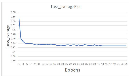
図4. 損失関数の値の変化.
