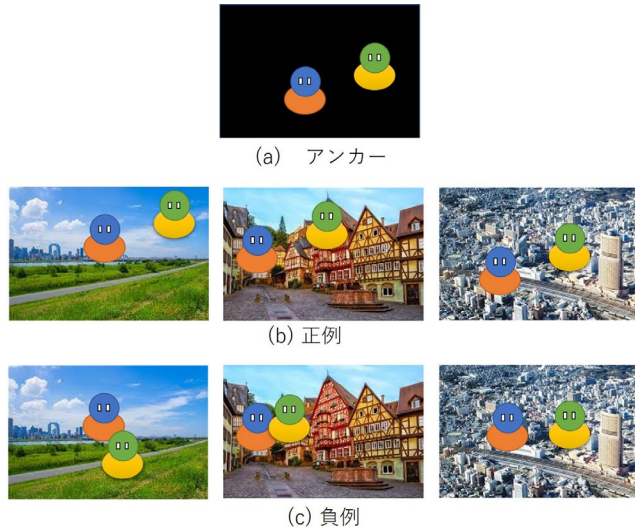
図2. Supervised Contrastive Learningにおけるアンカー画像(a)とそれに対する正例(b)と負例(c)。
